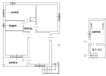
PIANTA PIANO TERRA H = m. 2.70
